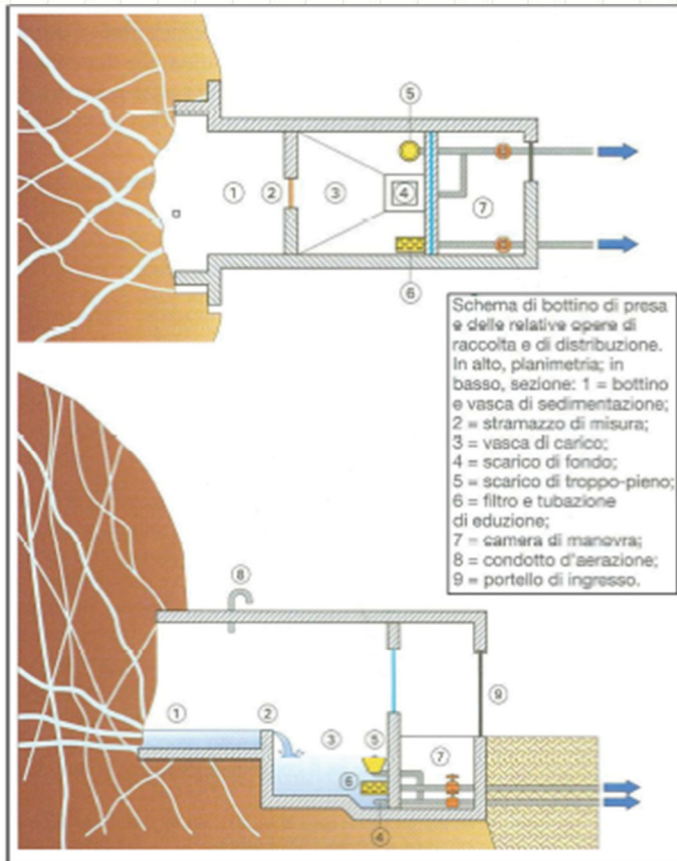
Figura 3 - Schema del bottino di presa (Civita. 2005)
