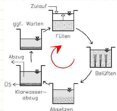
Abbildung 112: Prozessphasen beim SBR-Betrieb
