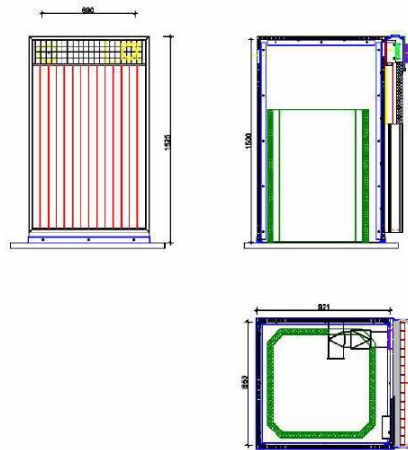
Abbildung 102: Abmessungen Solarkomposter mit Ansicht, Längs- und Querschnitt
