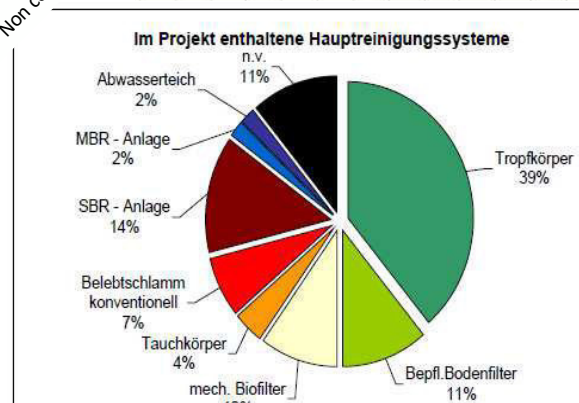
Abbildung 113: Im Projekt enthaltene Hauptreinigungssysteme
