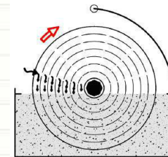
Abbildung 109: Schema Rotationsstaukörper
