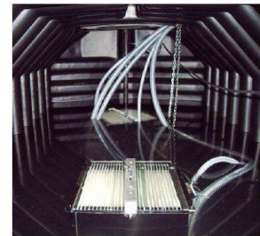
Behälter der Kläranlage im Technikraum der Olpererhütte (links) Membranmodul im MBR-Tank bei Inbetriebnahme in Reinwasser (rechts)
