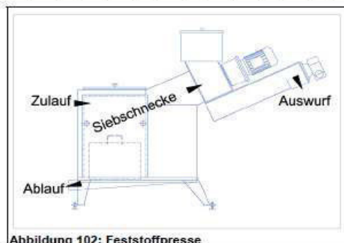
Abbildung 102: Feststoffpresse
